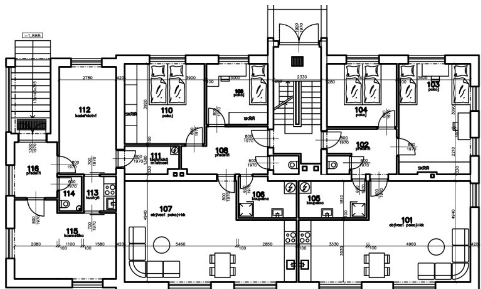
Plánovaná dispozície 1. NP objektu č. p. 120
